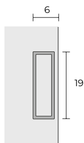
maniglia incassata inset handle
